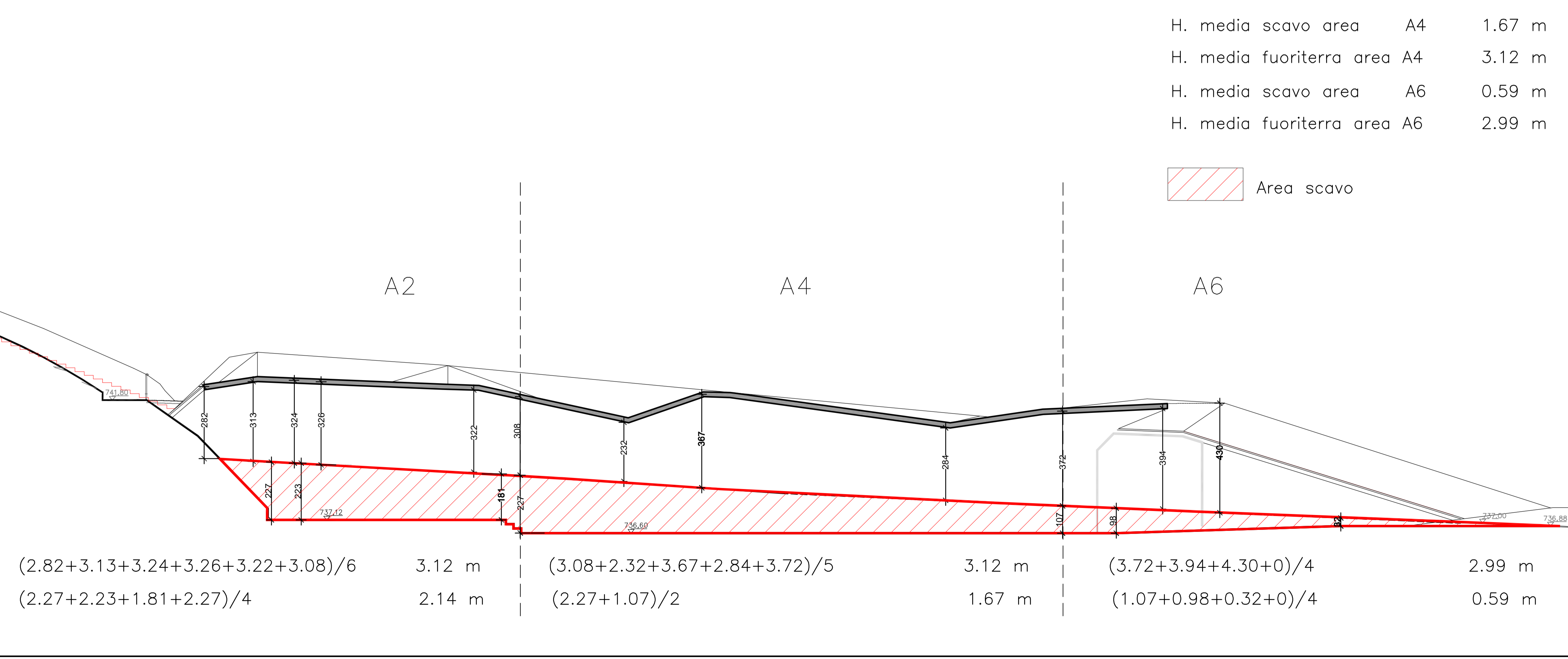
SEZIONE AA'
