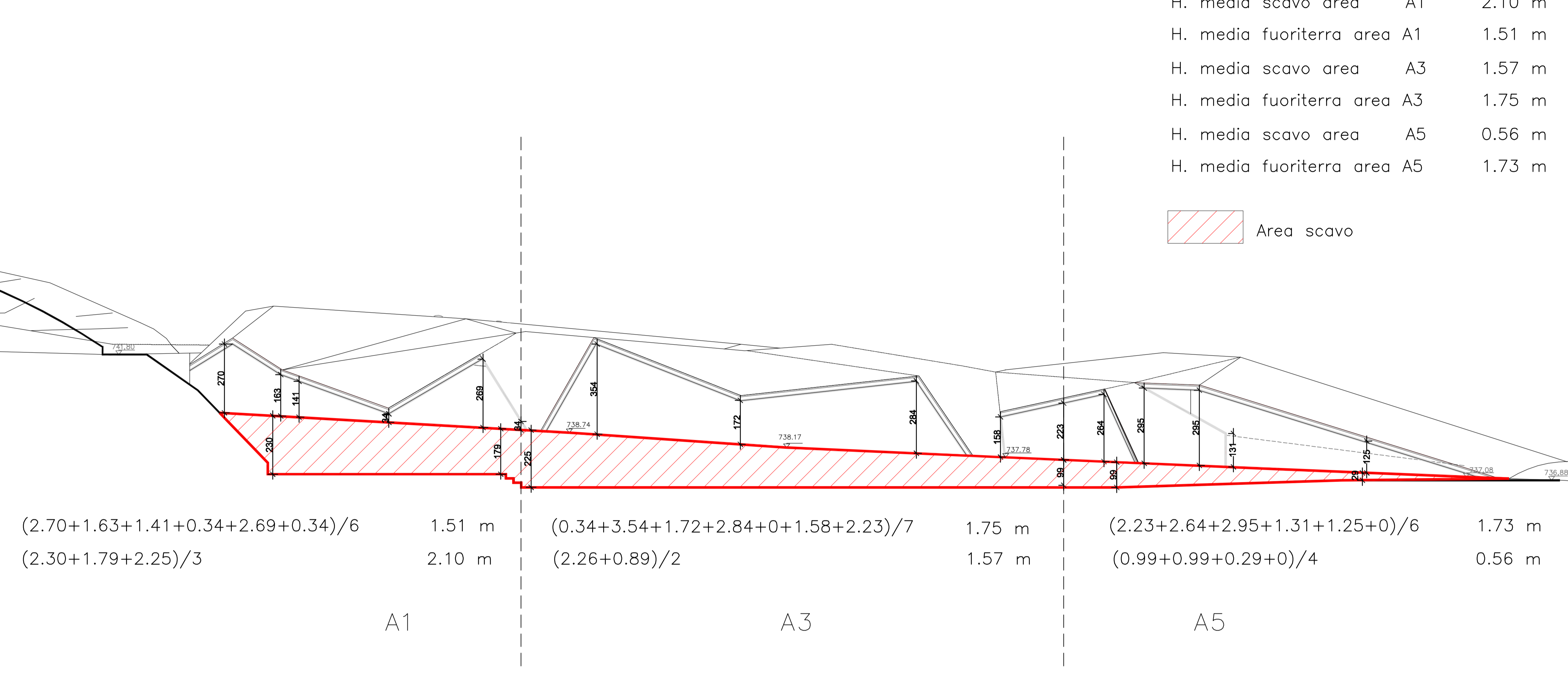
Sezione BB'
